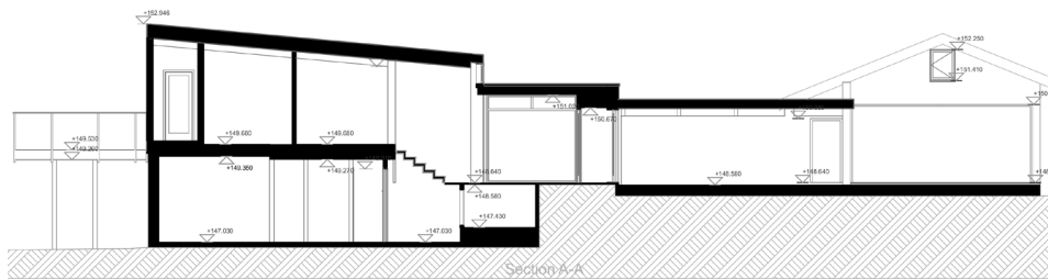
SCHNITT
