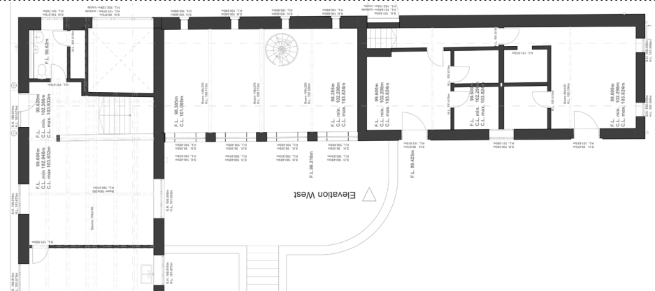
GRUNDRISS
